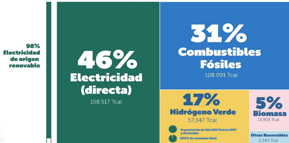
Figura 4: Consumo Final de Energía en Chile, 2050. PELP: Escenario Transición Acelerada: 345.205 Tcal.
