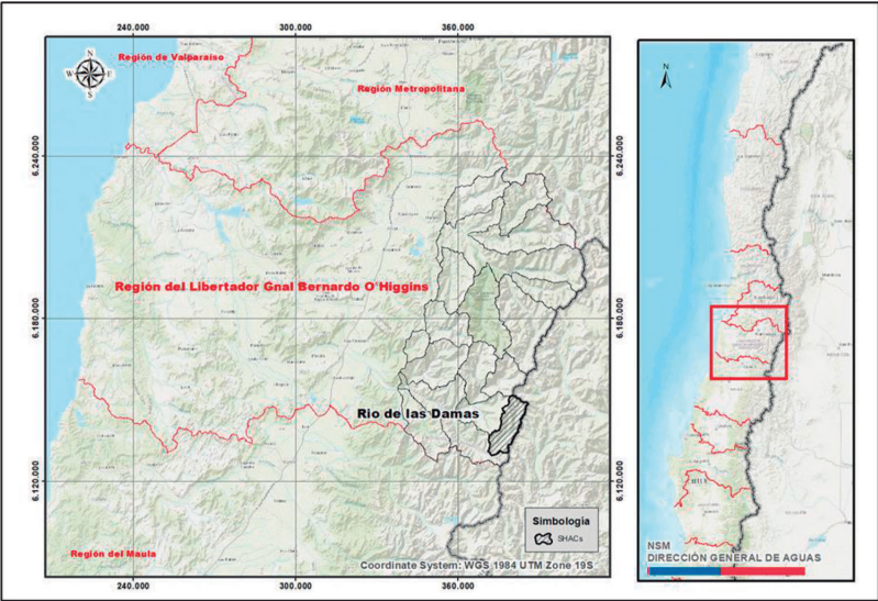
Mapa N° 1. Ubicación Sector Hidrogeológico de Aprovechamiento Común Río de las Damas
