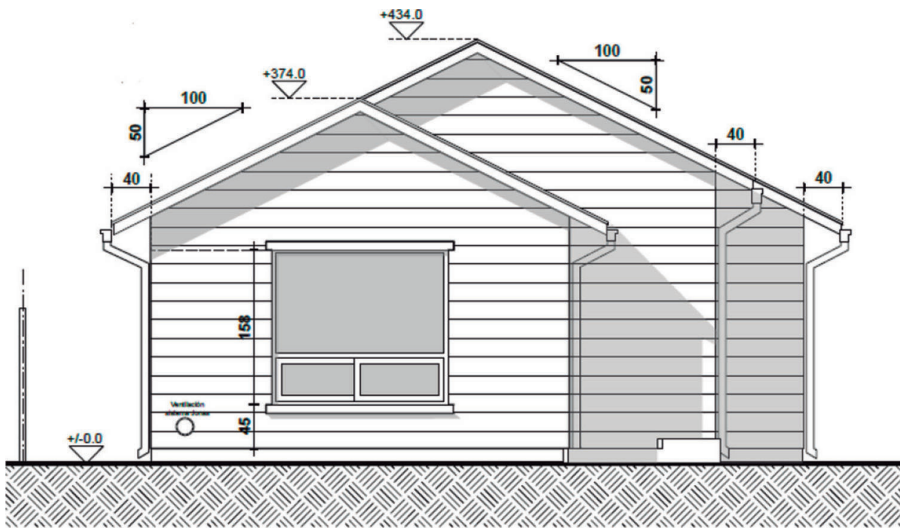
ELEVACION ANTERIOR esc. 1/50
