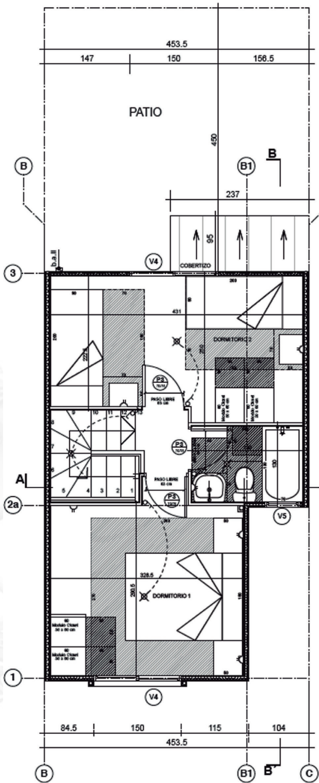
Planta Segundo Piso escala 1:50
