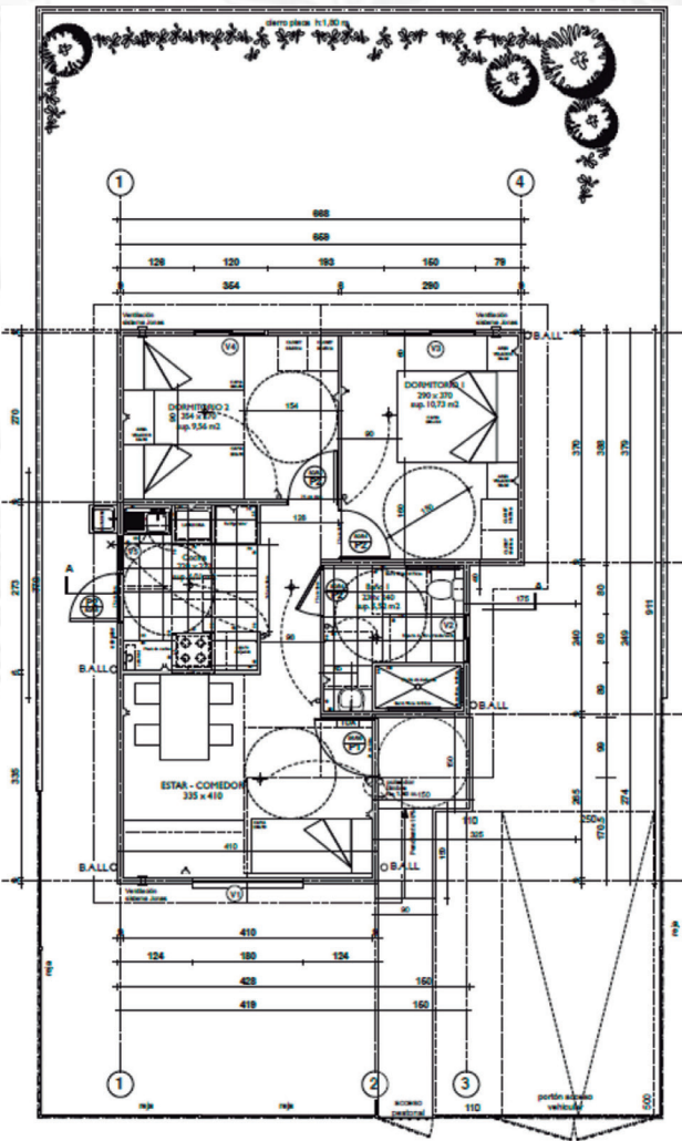
PLANTA esc. 1/50
